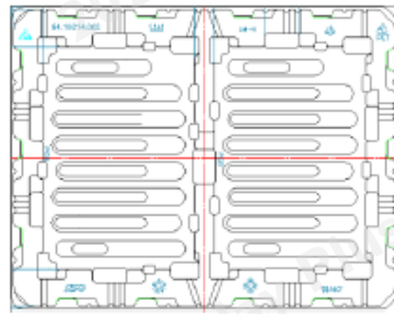
Tray 置放於 PP 瓦楞板上
