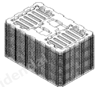
Tray 依上述方式依序正向堆疊，共堆疊 16+1 层 (Module 共 32 片，最上面第 17 个 tray 是空的)
